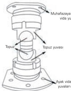
Muhafazaya sabitleme vida yuvası
