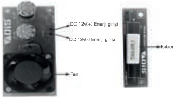
Isıtıcı + Soğutucu
