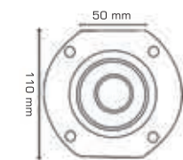
Muhafazaya sabitleme vida yuvası
