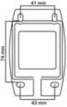
Muhafaza sabitleme vida yuvaları
