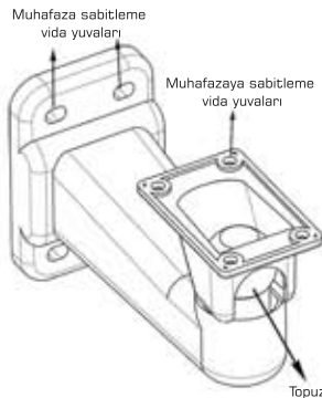
Muhafazaya sabitleme vida yuvaları
